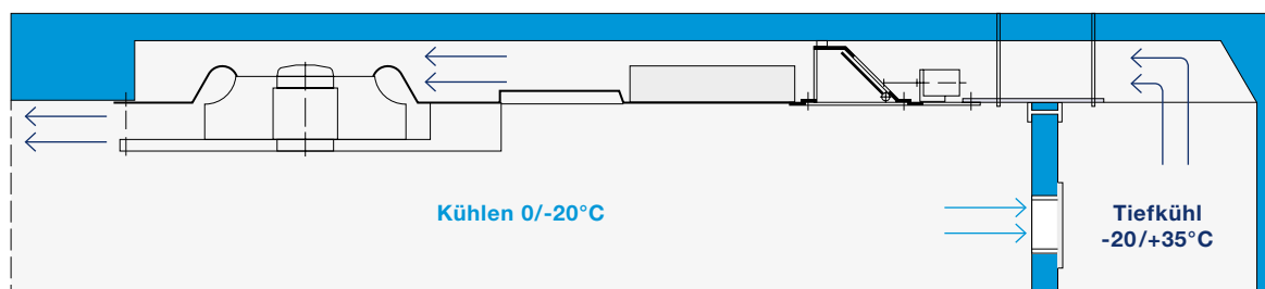
Deckenlüftersystem mit automatischer Heizung für Mehrkammerfahrzeuge
